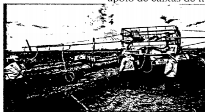
Carreta de apoio. Detalhes – tanque com gel, mangueiras para aplicação do gel, barra de apoio de caixas de mudas e equipe de plantio.
