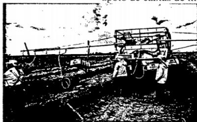
Carreta de apoio. Detalhes – tanque com gel, mangueiras para aplicação do gel, barra de apoio de caixas de mudas e equipe de plantio.
