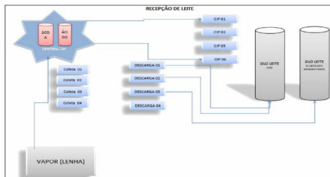
Figura 3 – Fluxograma do recebimento do leite cru
