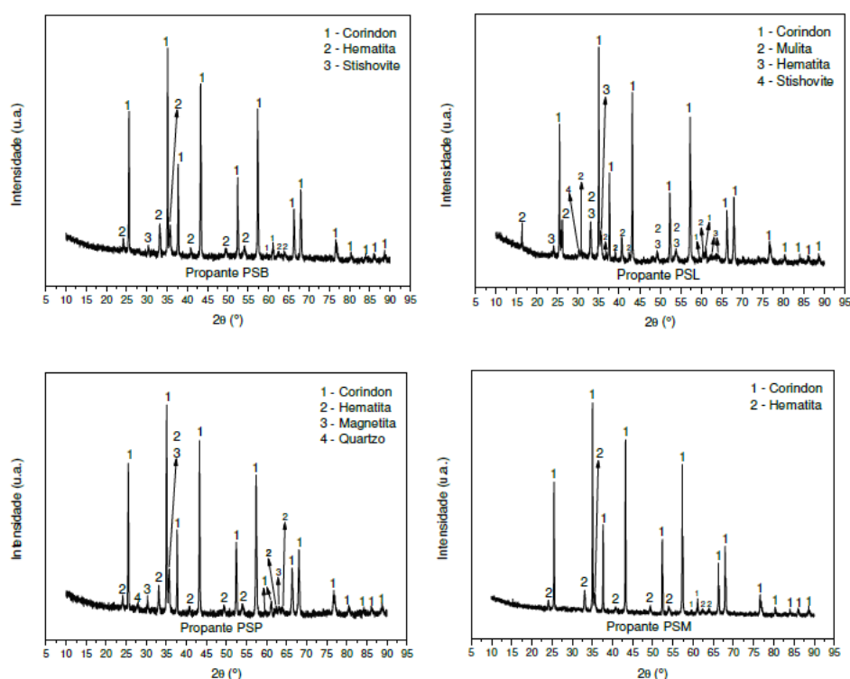
Figura 21. Difratograma de raios X dos propantes cerâmicos evidenciando a formação de corundum.
